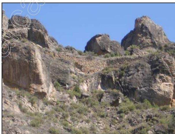
Figura 1: rocas carbonatadas
